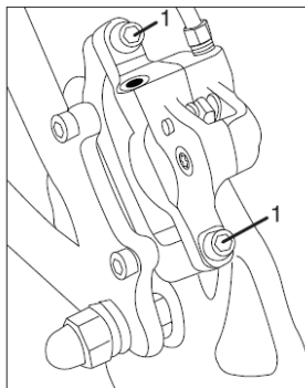
1. Регулировочные винты
