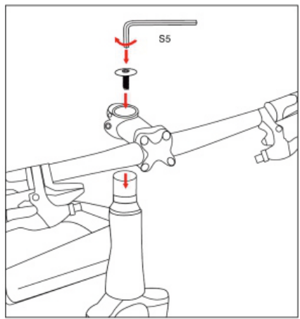
1. Снимите верхний винт штока вилки.
